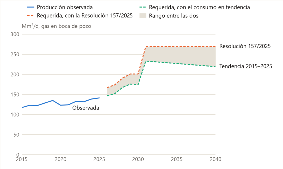
井口天然气产量，单位为百万m 3 /日：2015–2025年为观测值；2026–2040年为所需产量，分别按Resolución 157/2025（第157/2025号决议）设定的消费量和趋势消费量计算。两条路径均计入SESA的浮式液化天然气装置，并自2031年起计入Argentina LNG第一阶段■ 39 。图中文字为西班牙文。
