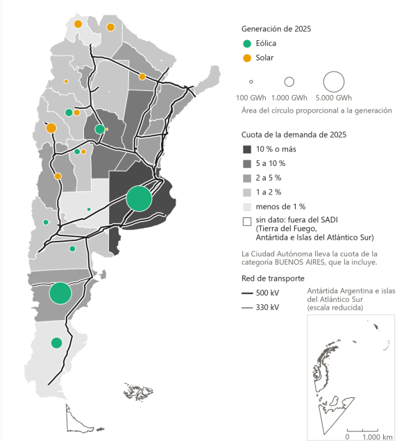
图：500 kV输电网络、风电场和光伏电站，以及2025年按CMMESA区域类别划分的电力需求 ■33 。图中文字为西班牙文。
